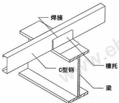
C型钢安装示意图
